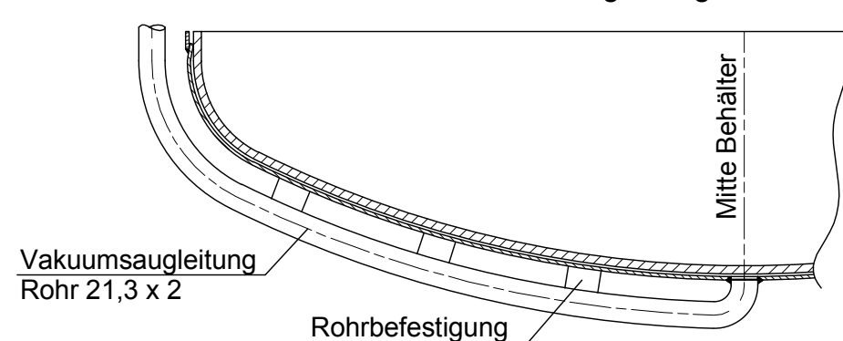
Detail "U" - Anschluss Vakuumsaugleitung -
