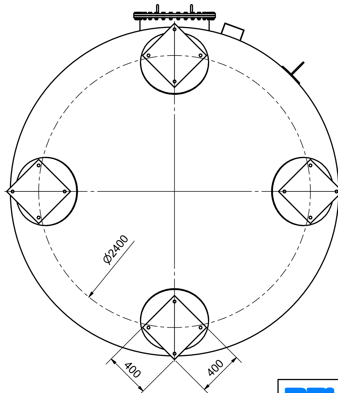
Ansicht von unten ( 1 : 20 )
