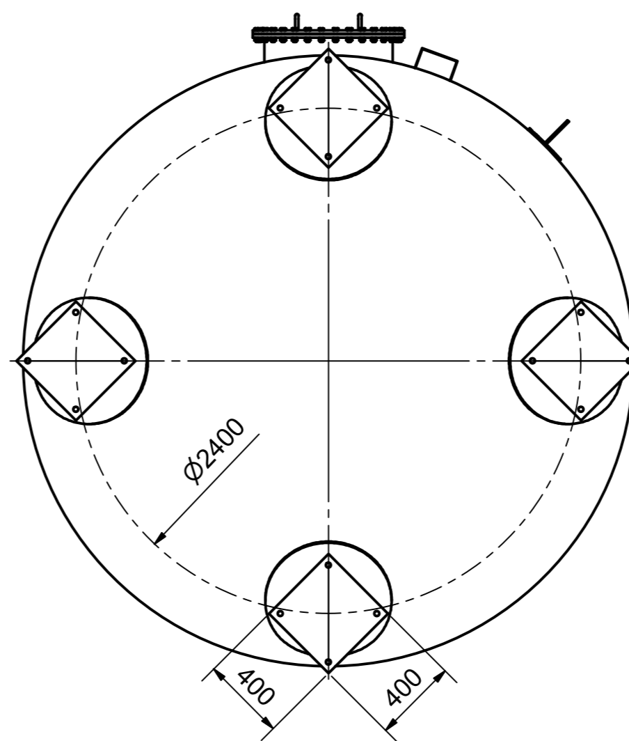
Ansicht von unten ( 1 : 25 )
