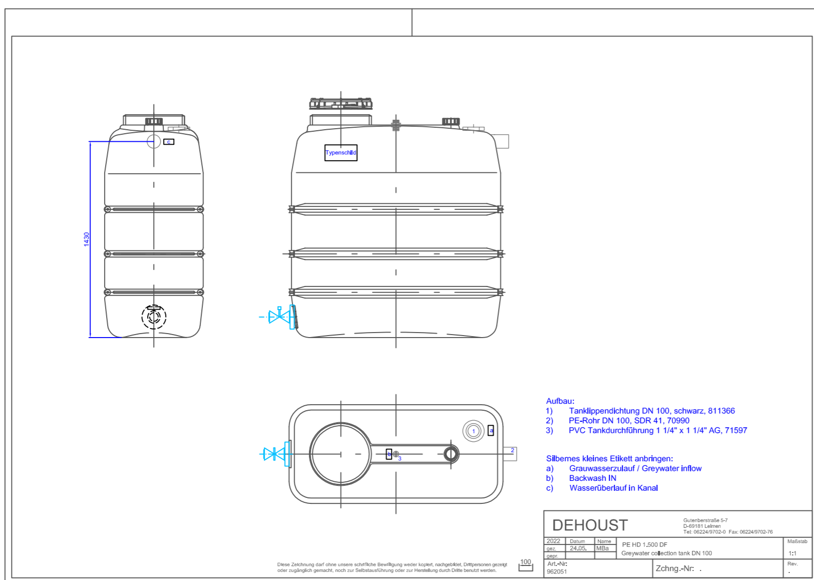
Greywater collection tank PE HD 1.500 DF
