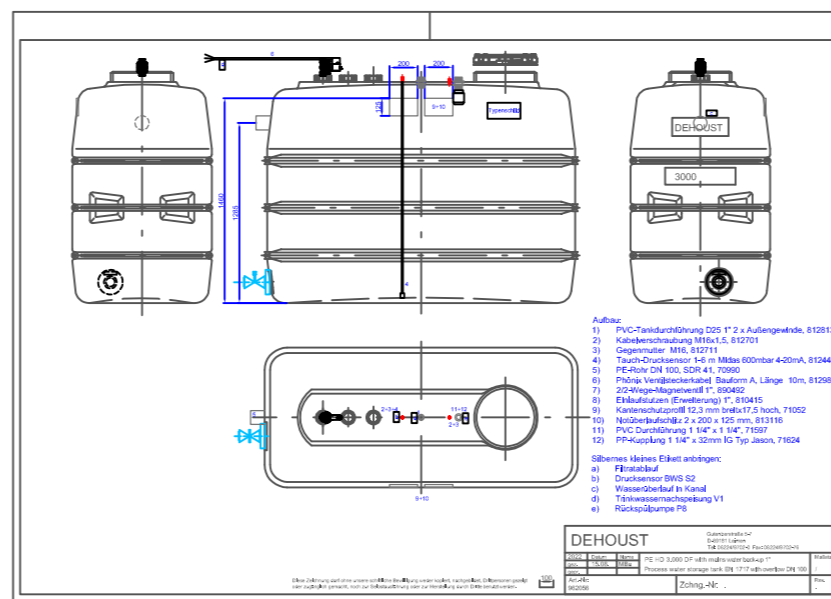
Process water storage tank PE HD 3.000 DF
