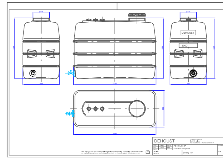
Extension storage tank PE HD 3.000 DF
