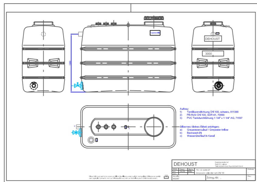
Greywater collection tank PE HD 3.000 DF
