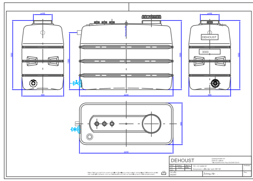
Greywater collection tank PE HD 3.000 DF
