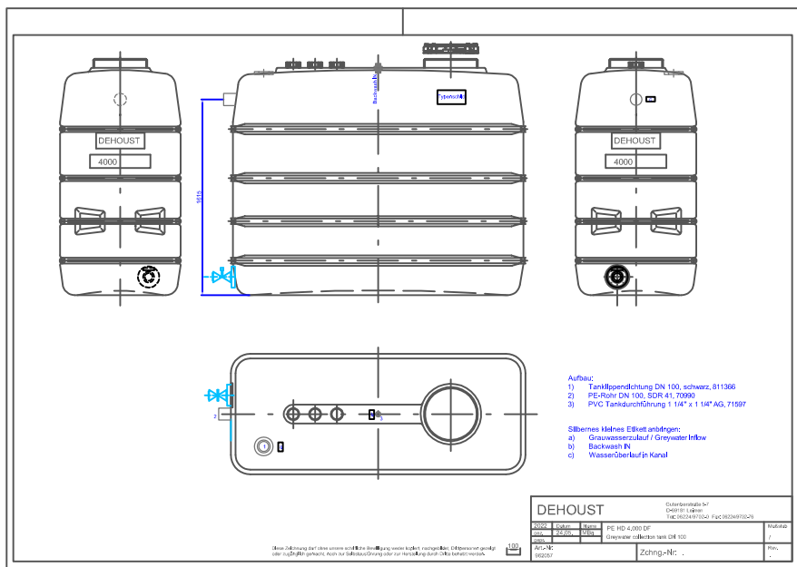
Greywater collection tank PE HD 4.000 DF
