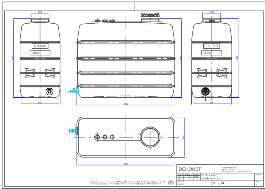
Extension storage tank PE HD 4.000 DF
