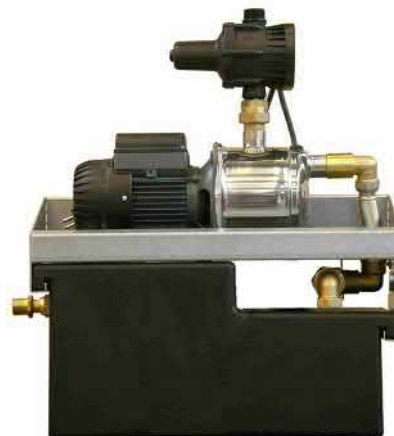
Sicherheitstrennstation ST5 ohne Haube
