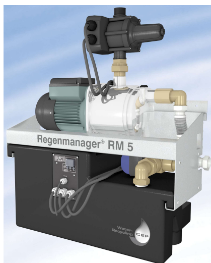
RM5 Plus Innenansicht
