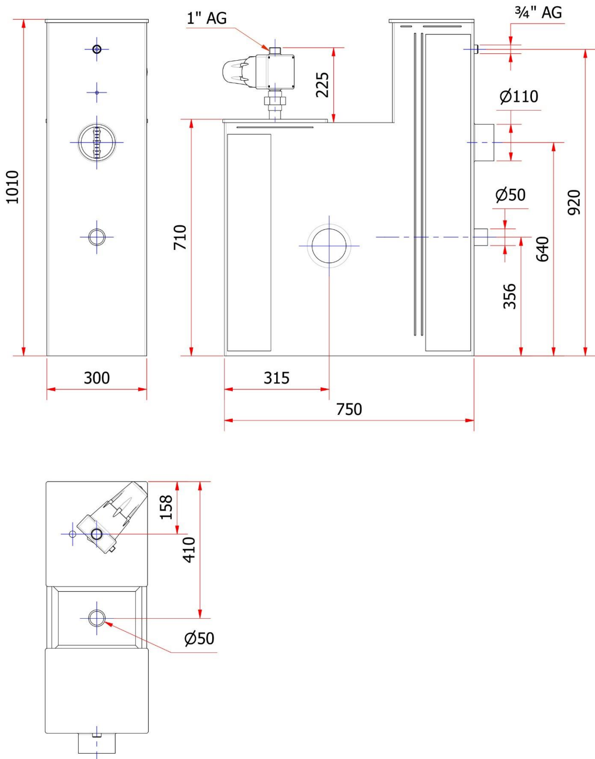
Abbildung 4: Abmessungen
