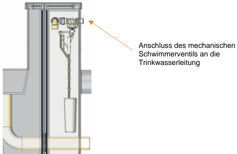
Abbildung 6: Anschluss der Trinkwassernachspeisung
