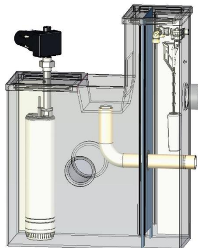
Abbildung 5: Tauchdruckpumpe mit DIGIMATIC im Vorratsbehälter
