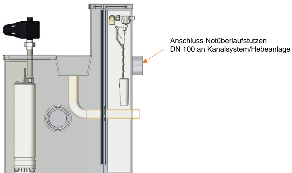
Abbildung 8: Anschluss des Notüberlaufstutzens
