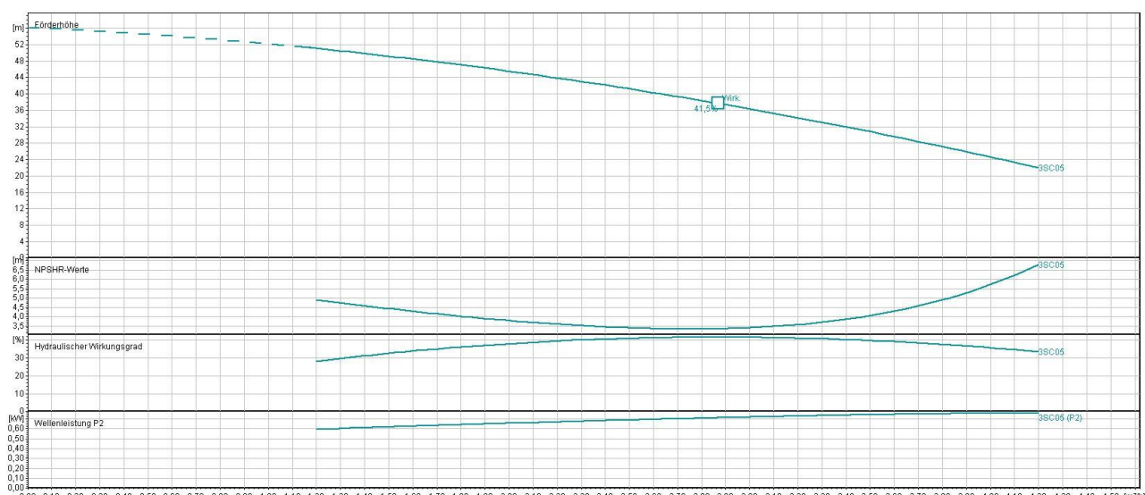
Abbildung 2: Pumpenkennlinie der Sicherheitstrennstation ST 5-4,35
