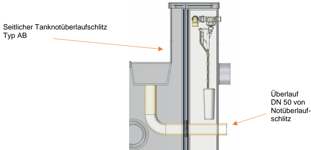
Abbildung 9: seitlicher Tanknotüberlaufschlitz Typ AB
