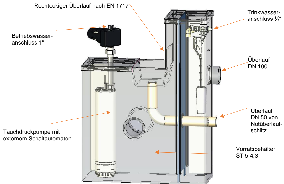
Abbildung 3: Aufbau der Sicherheitstrennstation: Vorderseite
