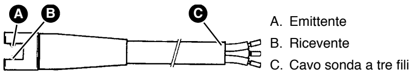
Figura 1: Sonda fotoelettrica
