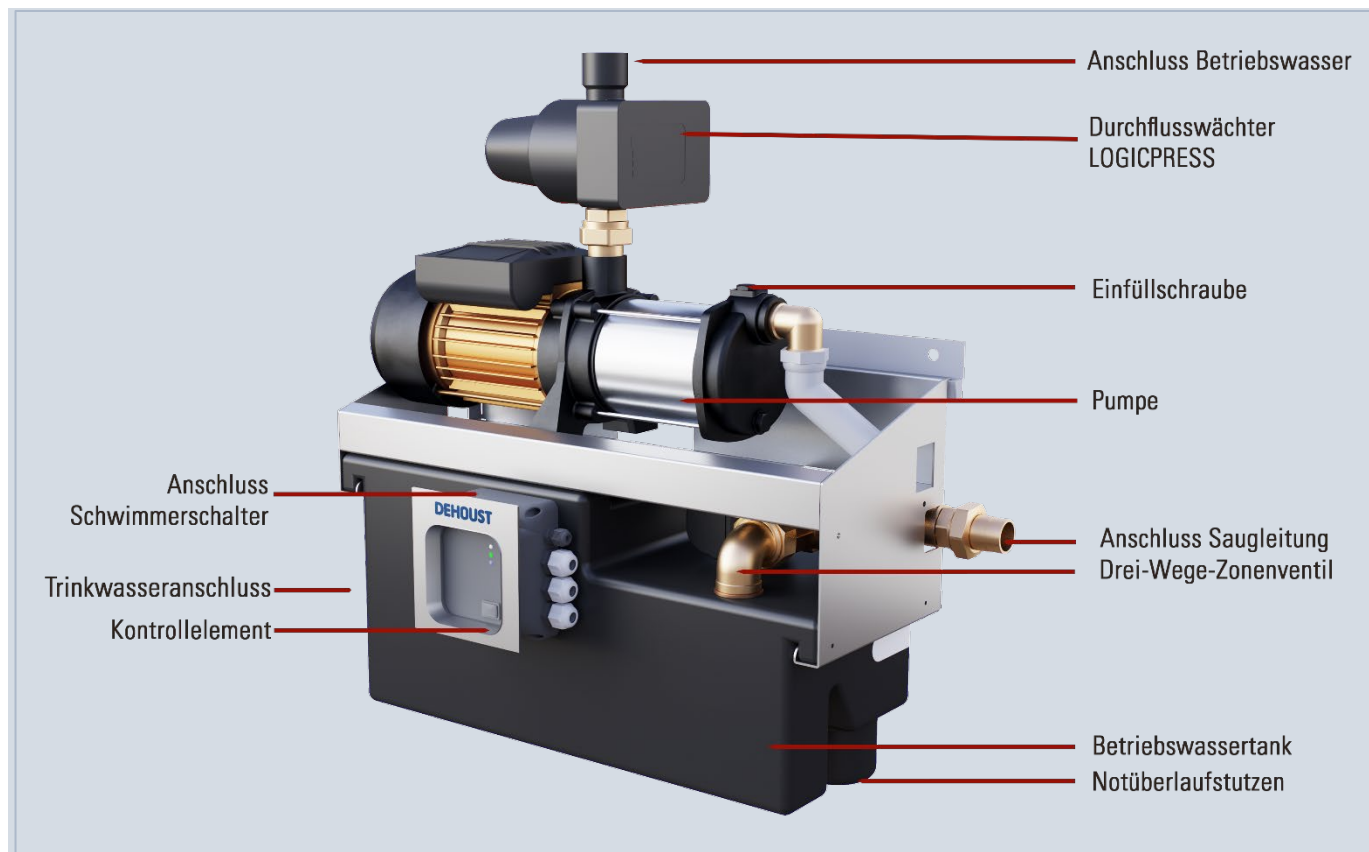
Abbildung 1: Regenmanager® RM5 Legende
