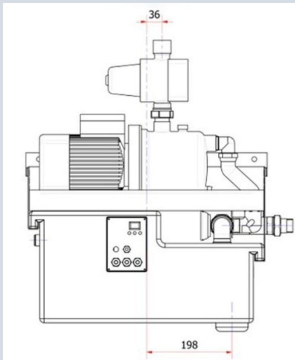
Abbildung 3: Anschlussmaße
