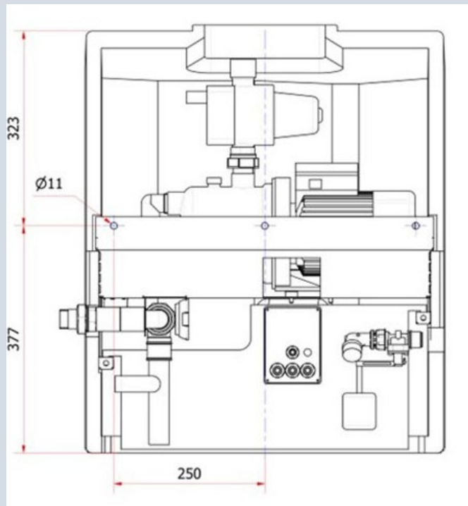
Wandhalterung hinten
