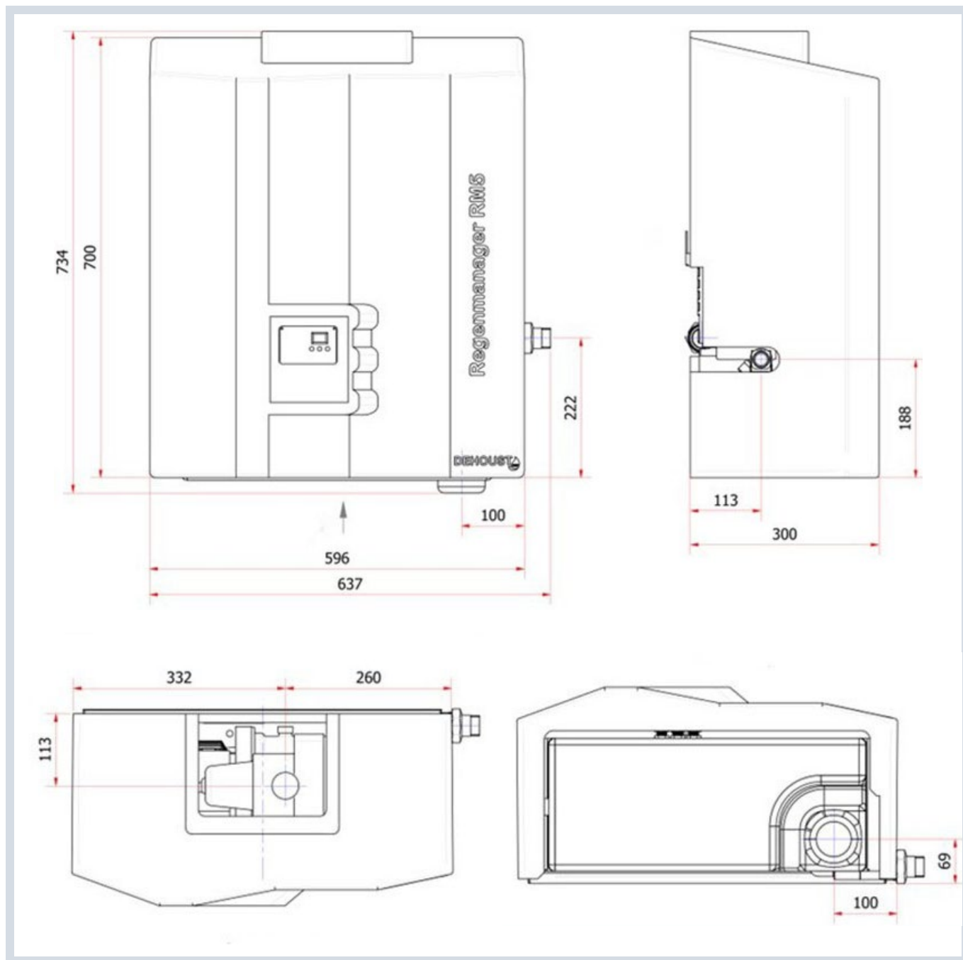
Abbildung 2: Außenmaße
