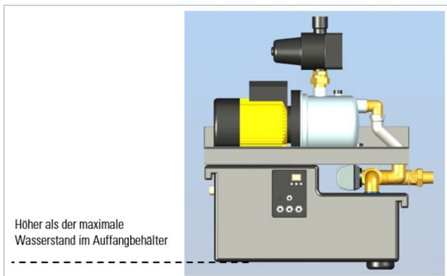
Abbildung 5: Rückstauenebene
