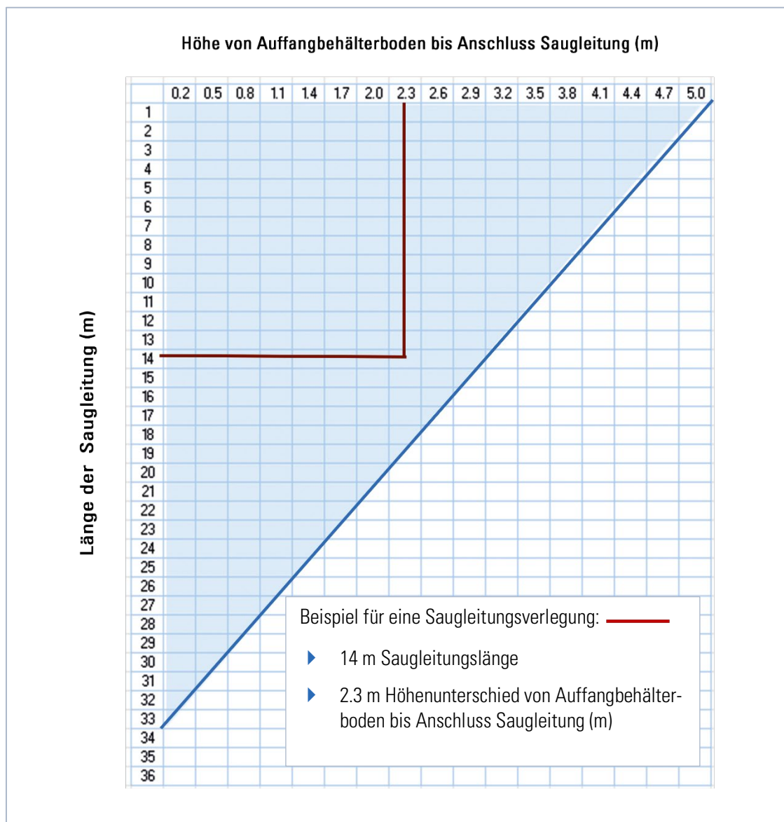
Abbildung 7: Darstellung Verhältnis Länge der Saugleitung zu Höhe vom Auffangbehälterboden (z. B. Zisterne/ Erdbehälter) bis Anschluss-Saugleitung; Bemessungsgrundlage der Tabelle: 1"PE-Saugleitung (25 mm Innendurchmesser) bei einem verbraucherbedingten Spitzendurchfluss von max. 5 m³/h.
