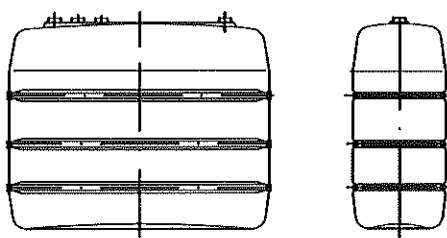
2.000 l - 2500 l - 3000 l mit 3 Bandagen
