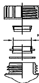
Detail - Stutzen
